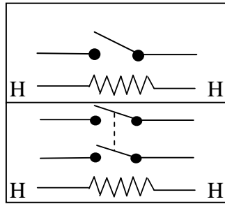
EKS-031 SPST+DPST Switch
