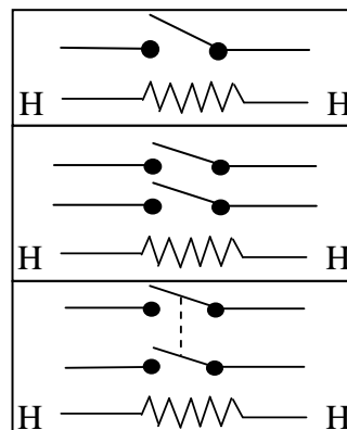
EKS-033 SPST+2SPST+DPST Switch
