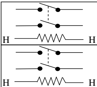
EKS-032 DPST+DSPST Switch
