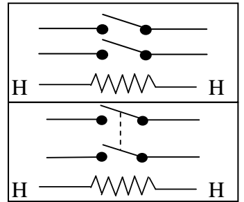
EKS-032 2SPST+DPST Switch
