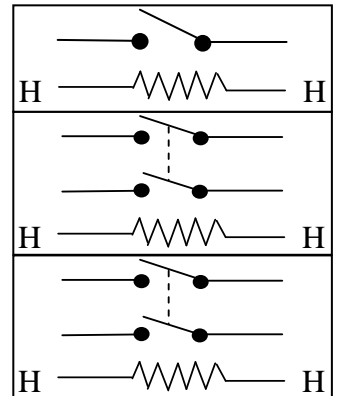
EKS-033 SPST+DPST+DPST Switch
